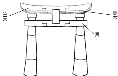
▶肥前鳥居の構造
